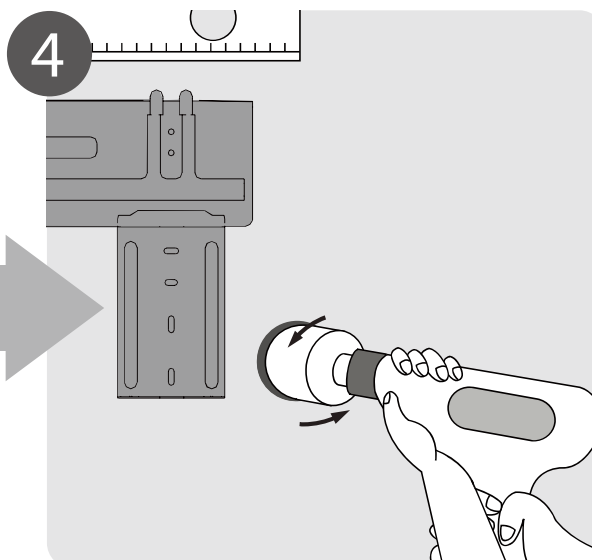
4 Perforar la pared (Página 12)
