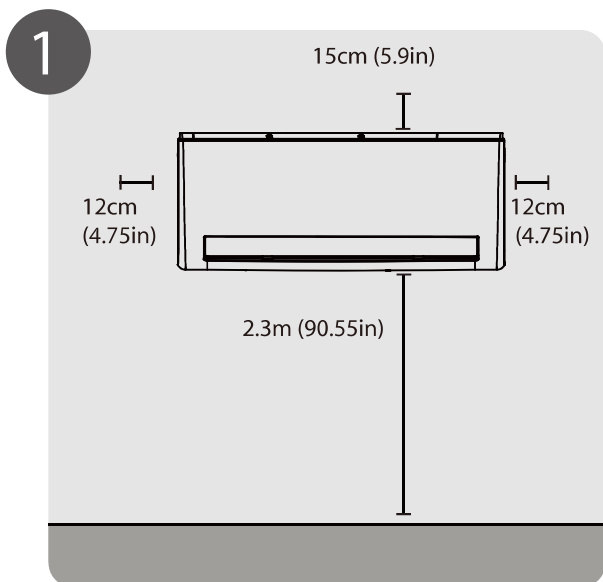
1 Seleccionar el lugar de instalación (Página 11)
