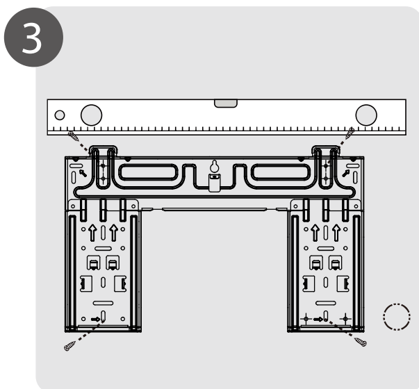
3 Instalar la base de montaje (Página 12)
