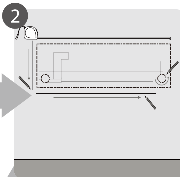
2 Determinar el lugar de la perforación (Página 12)
