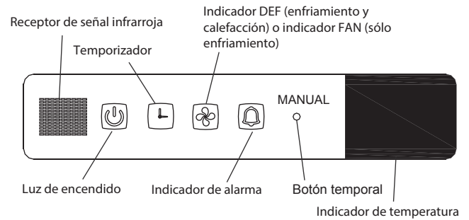
Panel del Display fig. 2-2
