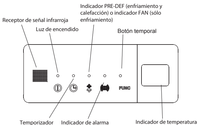
Panel del Display fig. 2-8
