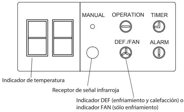
Panel del Display fig. 2-4
