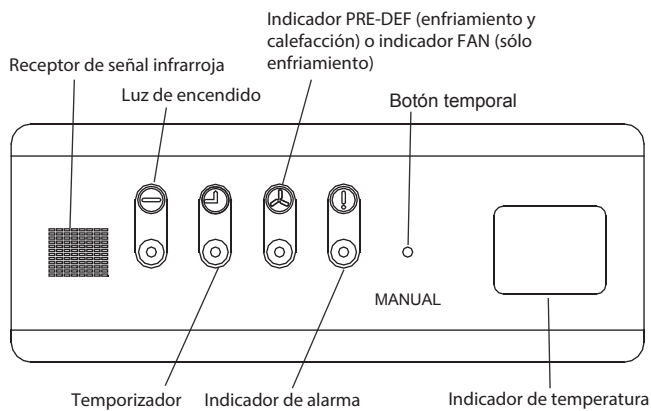
Panel del Display fig. 2-7
