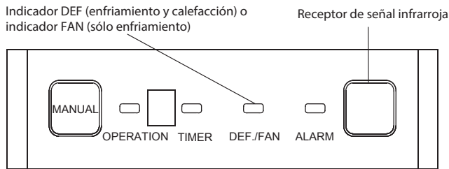
Panel del Display fig. 2-5
