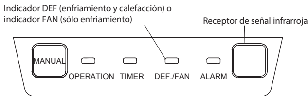
Panel del Display fig. 2-6
